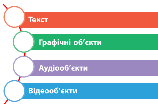
Рис. 1. Об'єкти мультимедіа
