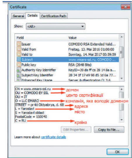
Рис. 4. Вкладка Details
