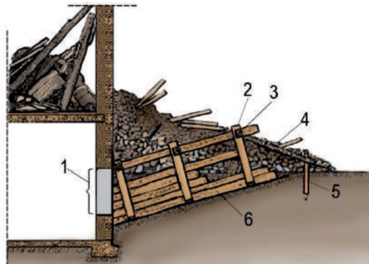
Іл. 34.10. Траншея в уламках: 1 — стіновий пролом; 2 — брус для перекриття; 3 — розпірка; 4 — розкіс; 5 — паля для закріплення; 6 — дошки обшивки
